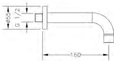
Ref.: 68911 45 Box: 1 | Carton: 40 | Pallet: 640
