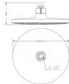
Ref.: R65112 18 Box: 1 | Carton: 24 | Pallet: 144
