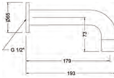
Ref.: 1668 41 Box: 1 | Carton: 21 | Pallet: 360
